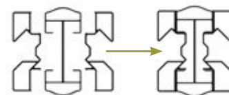
Composition du profil d'angle
